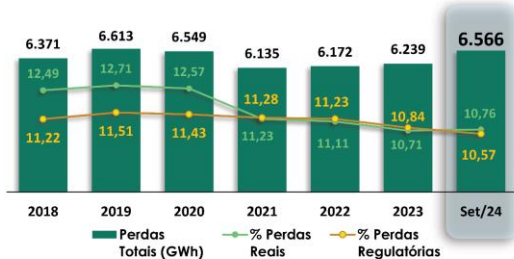
Perdas - Janela móvel de 12 meses
